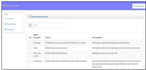
Gambar 4.4 Halaman Data Penyakit
